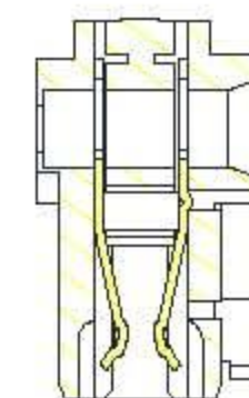
SECTION:B-B
